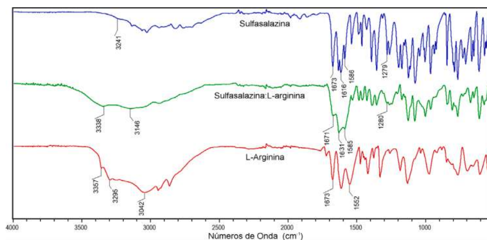
Figura 3. Espectros de FT-IR.
