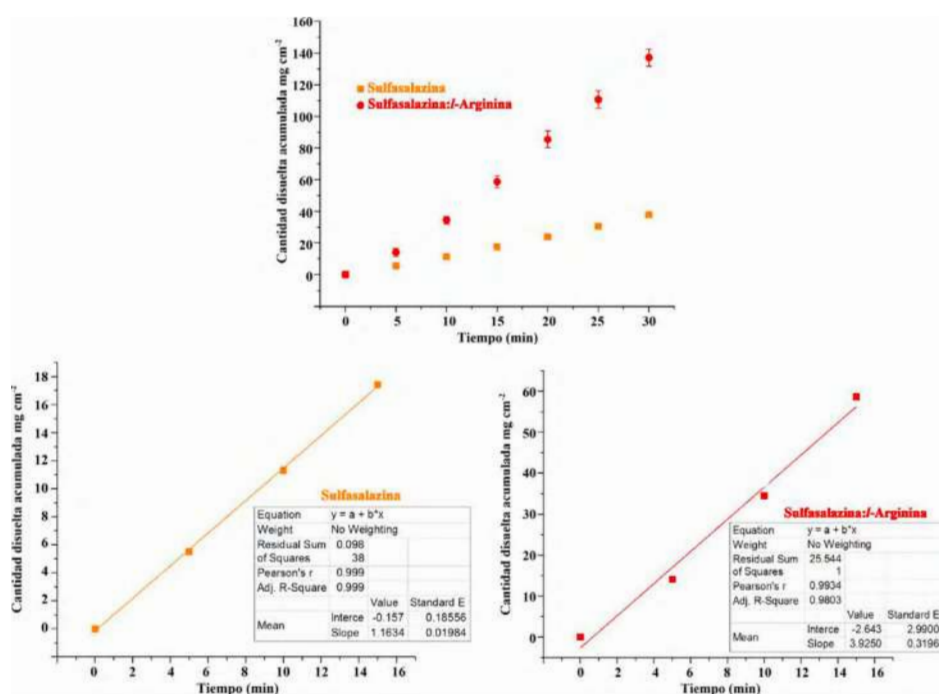
Figura 7. Gráfico de Arriba, velocidad de disolución a pH 6.8 a 37^\circ\text{C} y 50 rpm. Gráficos de abajo, cálculos de la constante de disolución de Sulfasalazina y el co-amorfo sulfasalazina L -Arginina.
