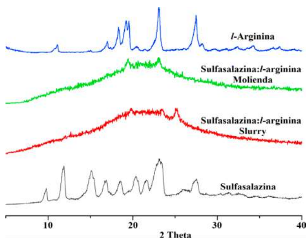
Figura 2. Difractogramas de Rayos X de polvos.
