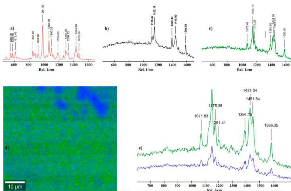
Figura 4. Espectros de microscopía Raman de: a) L-Arginina y b) Sulfasalazina y c) de la fase co-amorfa obtenida; abajo, d) imagen obtenida mapeo y e) espectros que corresponden a las zonas verde y azul de la imagen de mapeo.
