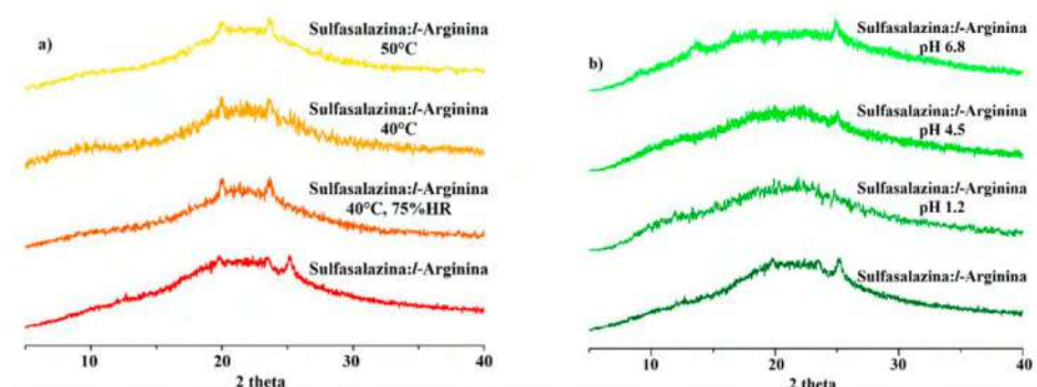
Figura 6. Difractogramas de rayos X de polvos de a) prueba de estabilidad indicativa del co-amorfo bajo diferentes condiciones de temperatura y HR y b) Prueba de estabilidad del co-amorfo a diferentes sometido 24h a diferentes medios fisiológicos al pH indicado.
