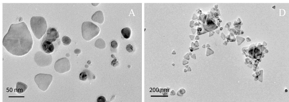
Figura 1. Imágenes de soluciones coloidales que contienen nanopartículas de plata sintetizadas con 1.2 (A), 0.9 (B), 0.6 (C) y 0.3 mL (D) de \text{NaBH}_4 .
