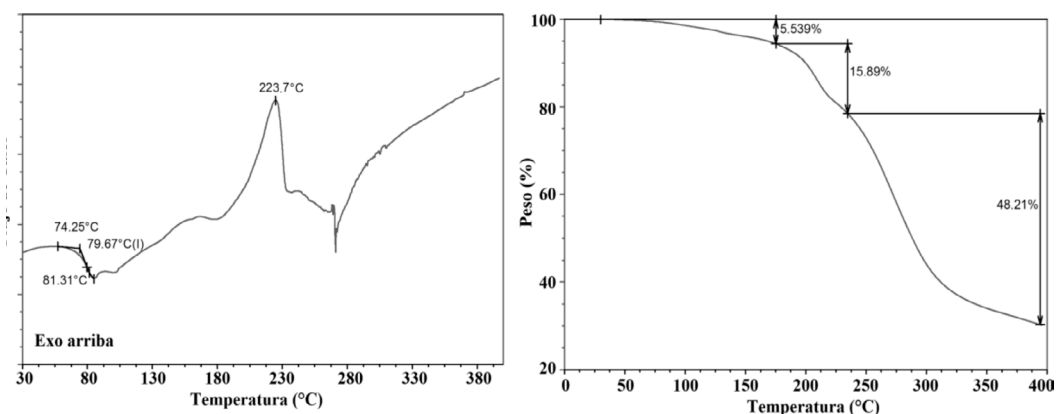
Figura 5. Termogramas de calorimetría de barrido diferencia DSC (a) y el análisis termogravimétrico TGA (b) de la nueva forma solida 1:1 Sulfasalazina:L-Arginina.
