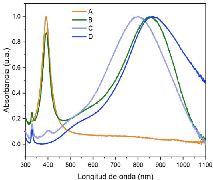
Figura 3. Espectros de absorbancia de soluciones coloidales que contienen nanopartículas de plata sintetizadas con 1.2 (A), 0.9 (B), 0.6 (C) y 0.3 mL (D) de \text{NaBH}_4 .
