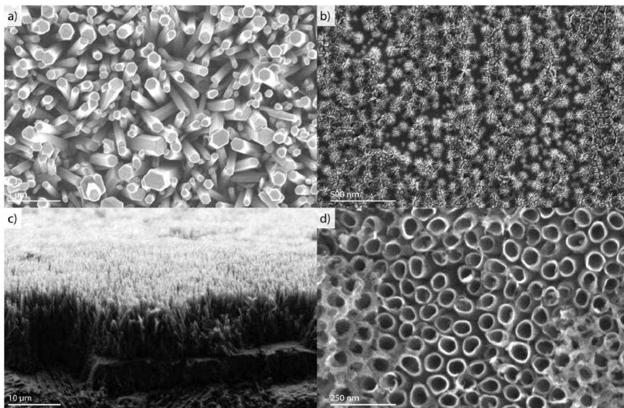
Figura 3. Morfologías nanométricas utilizadas para aumentar la efectividad de los sustratos SERS al incrementar notablemente el área superficial sobre la cual pueden depositarse las nanoestructuras plasmónicas. A) nanocolumnas, b) nanoflores, c) nanoalambres y d) nanotubos.
