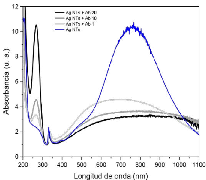
Figura 6. Absorbancia de soluciones con Ag NTs antes y después de incubar Ab CA19-9 con concentraciones de 1, 10 y 20 µg/mL.
