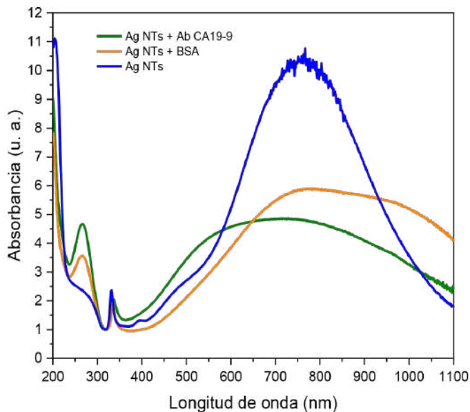
Figura 5. Espectros de absorbancia de soluciones de Ag NTs, Ag NTs con BSA y Ag NTs con Ab CA19-9.
