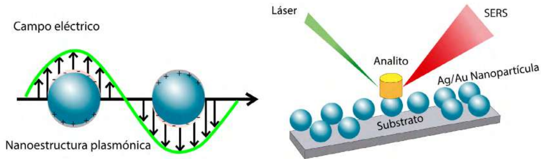
Figura 1. Principio SERS que utiliza nanoestructuras plasmónicas (nanopartículas) para amplificar las señales Raman.
